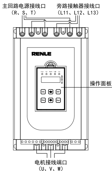
M1 主回路接线端口示意图
