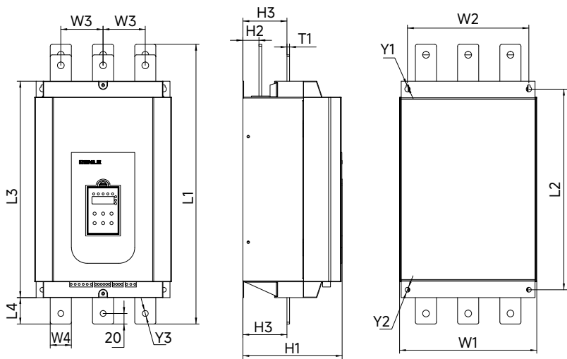
外形及安装尺寸表：
