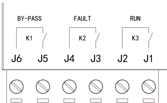
继电器端子接线图
